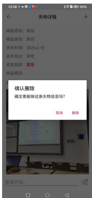
图 10-3 删除提示
