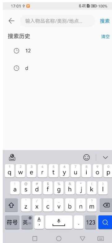
图 14 搜索页面
