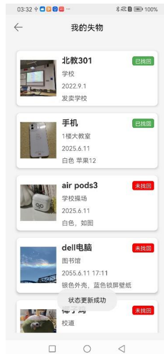
图 19-3 二次点击
