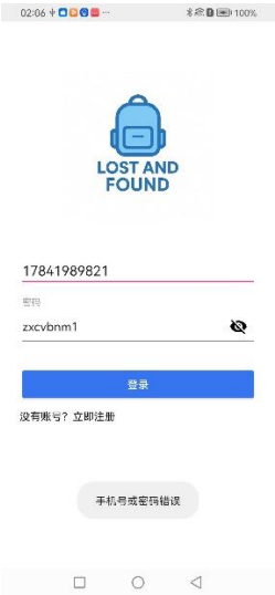
图 2-3 错误提示
